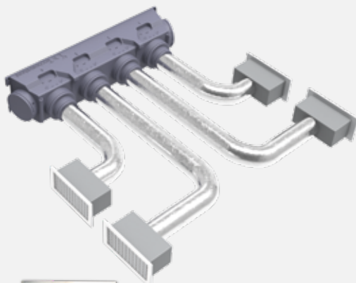
GRIGLIA DI RIPRESA CON FILTRO foro inst. 600 x 400mm
