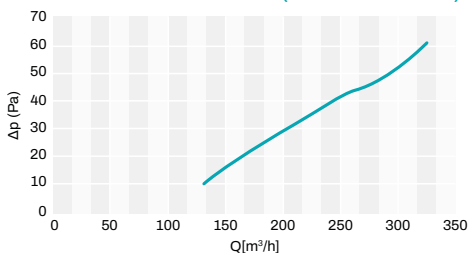
COLLO LATERALE DN. 100 mm (DIFF. 295 x 295 mm)
