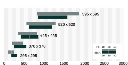
SELEZIONE RAPIDA PORTATA D'ARIA
