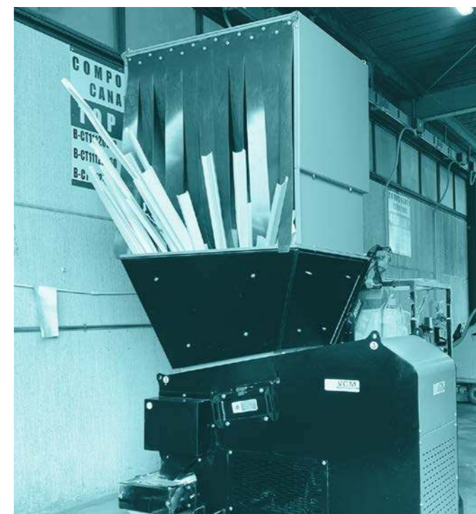
Mulino di macinatura del PVC scarto di produzione
