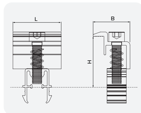
ABMESSUNGEN [mm]
