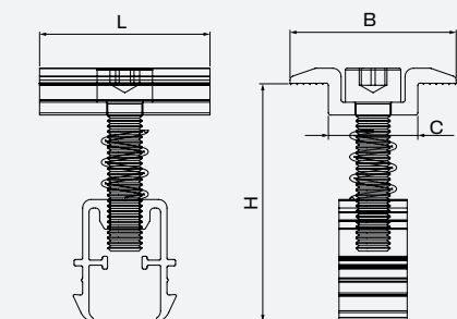
ABMESSUNGEN [mm]
