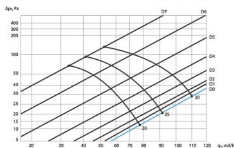
Canova Ø 125 (estrazione / exhaust air)
