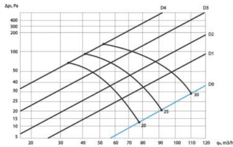
Canova Ø 100 (estrazione / exhaust air)
